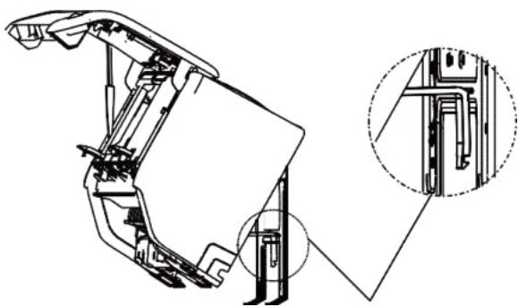
Használja a készülék hátulján lévő tartót az egység megtámasztásához
